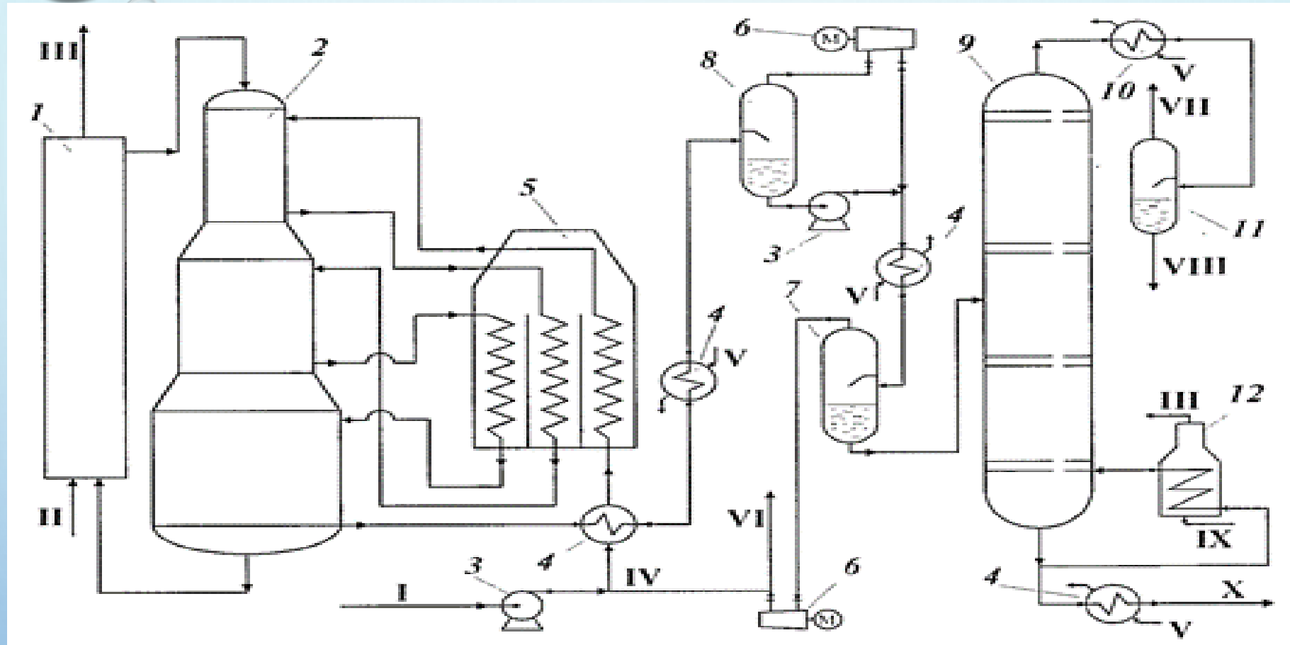
Сурет 1 - Қозғалмалы катализатор қабаты бар риформинг ондырғысының сызба-нұсқасы 1 - Регенерация секциясы; 2- реактор; 3-насос;4- жылуалмастырғыш; 5- көпсекциялы пеш; 6-компрессор; 7- жоғары қысымды газдысеператор; 8- төменгі қысымды газды сеператор; 9- тұрақтандыру колоннасы; 10- тоңазытқыш; 11- сеператор; 12- құбырлы пеш; I – шикізат; II – ауа; III – түтінді газдар; IV – циркулденетін газ; V – су; VI – сутек; VII – газтәрізді көмірсутектер; VIII – тұрақсыз фракция; IX – отынды газ; X – тұрақты катализат.
